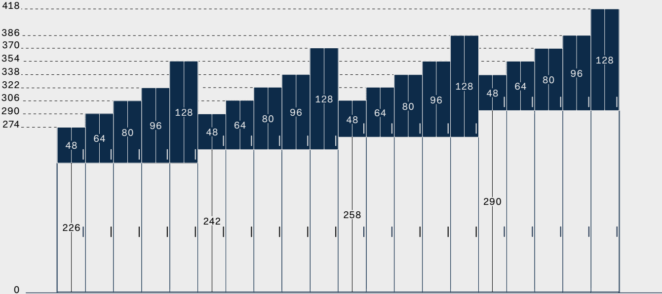
Altezze totali Total heights
