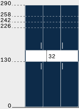
Nicchia H. 32 Recess H 32
