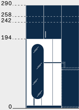
Nicchia con specchio Recess with mirror
